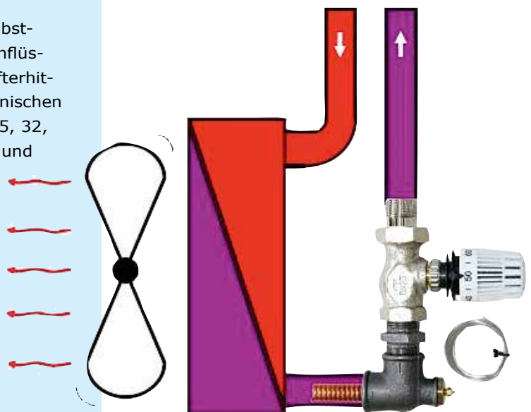
Einbaubeispiel RTB-Abgleich-Set an einem Lufterhitzer
