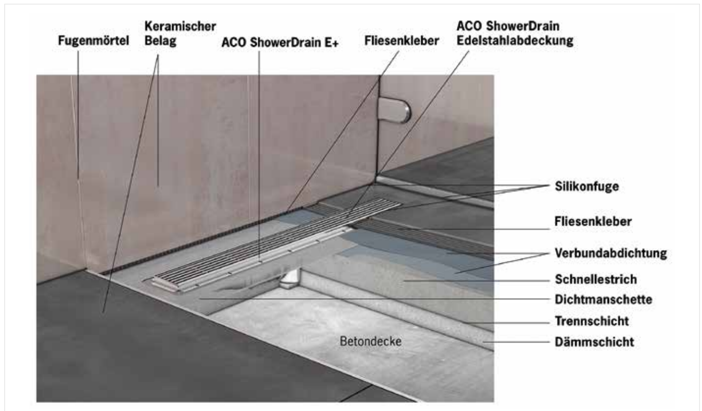
I Schematische Darstellung ACO ShowerDrain E+ mit Wandaufkantung mit Flüssigabdichtung.
