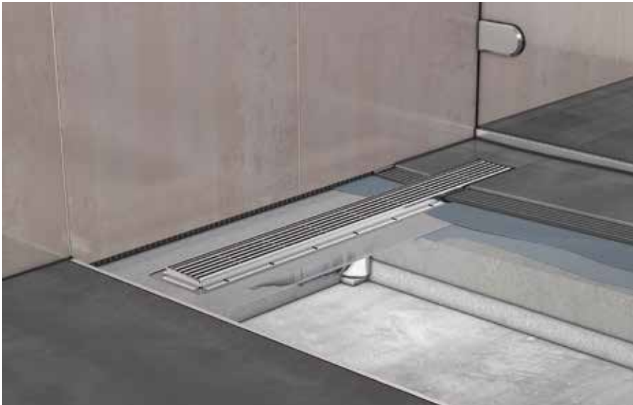
! Bodenaufbau eines barrierefreien Duschplatzes mit der neuen Edelstahl-Duschrinne ACO ShowerDrain E+.
