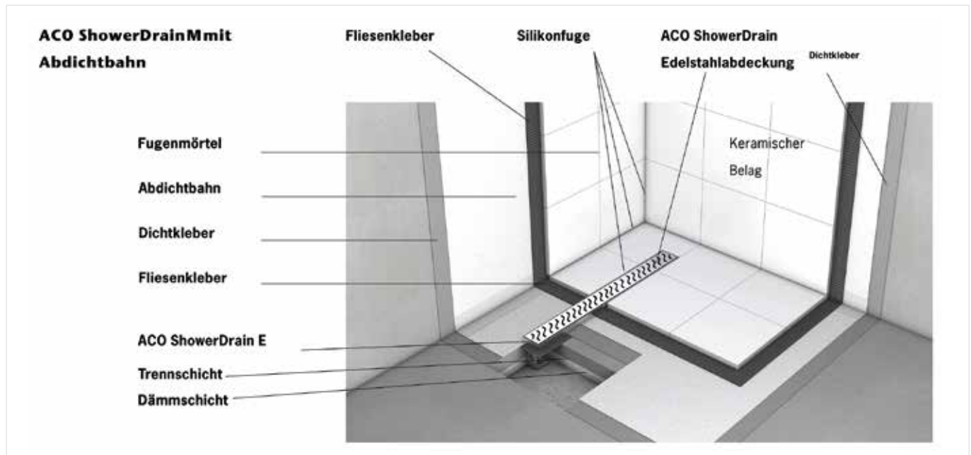
I Schematische Darstellung ACO ShowerDrain M+ mit Abdichtbahn.
